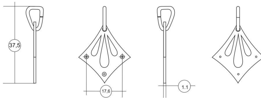
Рисунок 2. Пример технического рисунка ювелирного изделия «Кулон» Категория «Студенты»
